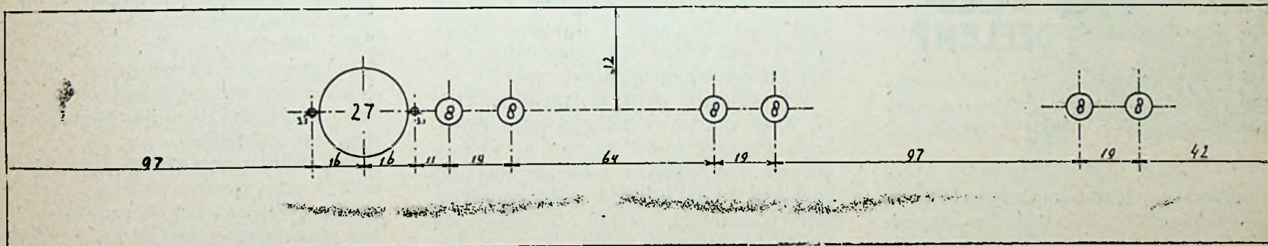
Fig. 4. Achterzijde chassis, \frac{1}{2} ware grootte.
