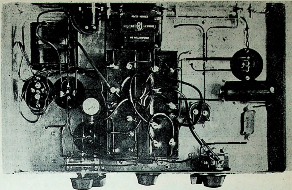
De onderzijde van het chassis.
