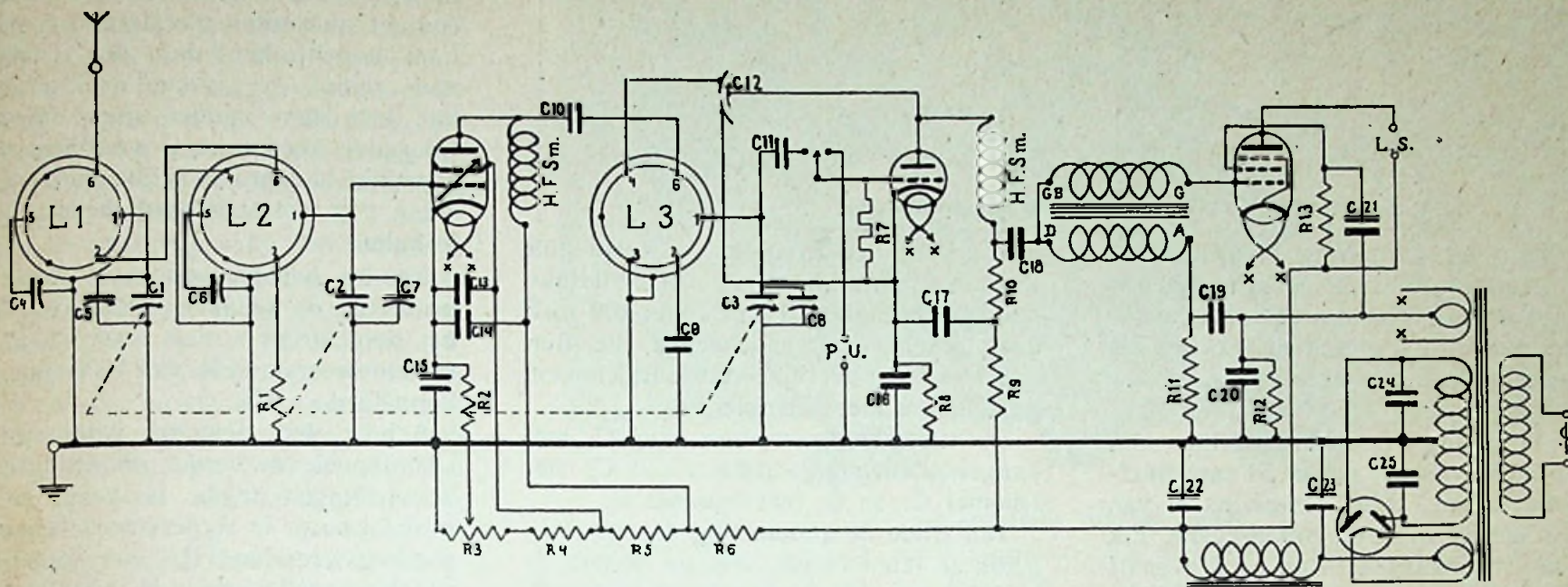
Fig. 1. Principe-schema.
